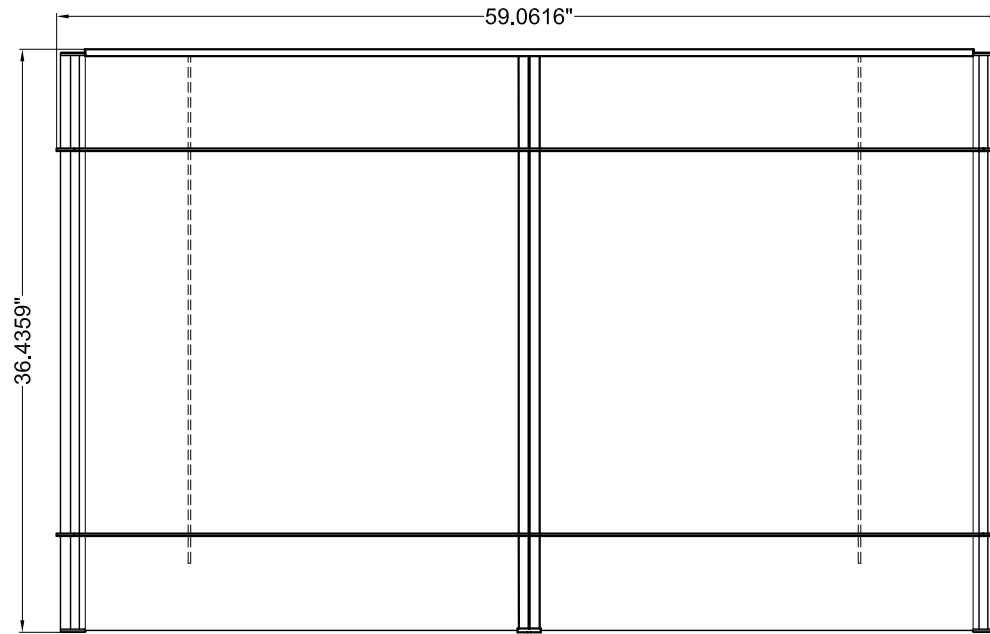
TOP ELEVATION
