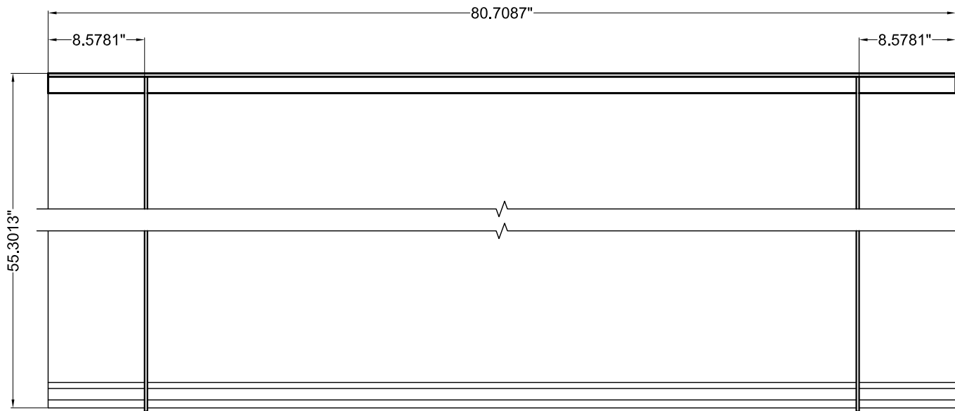
TOP ELEVATION
